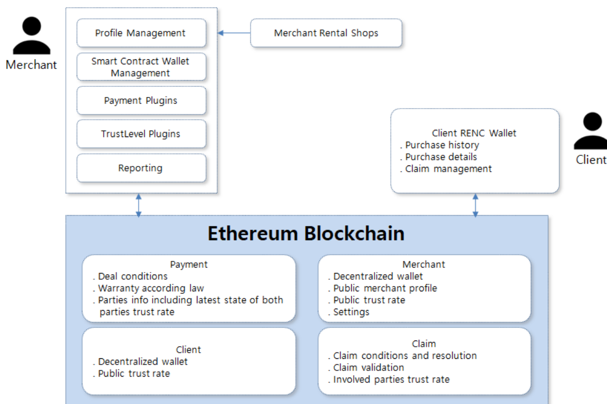
Hình 4, Kiến trúc RENC cho tiền tệ dịch vụ cho thuê
